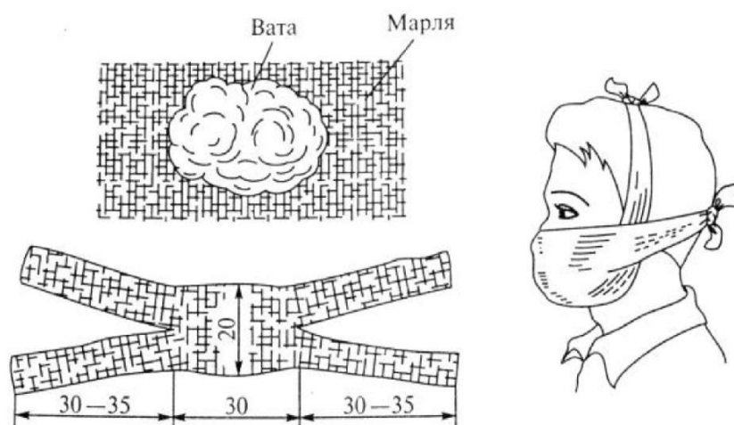
Рис. 5.14. Изготовление ватно-марлевой повязки (размеры в сантиметрах). К СИЗК относят защитную одежду фильтрующего и изолирующего типа. К изолирующим средствам защиты кожи относятся общевойсковой комплексный защитный костюм (ОКЗК), общевойсковой защитный комплект (ОЗК), легкий защитный костюм (Л-1), защитный комбинезон или костюм. Общевойсковой комплексный защитный костюм (ОЗК) предназначен для комплексной защиты от светового излучения и радиоактивной пыли, паров и аэрозолей ОВ и биологических аэрозолей. Он состоит из пропитанных специальным составом куртки, брюк, защитного белья, головного убора, подшлемника.
