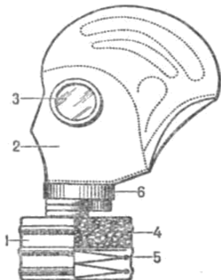
Рис. 1. Фильтрующий противогаз
