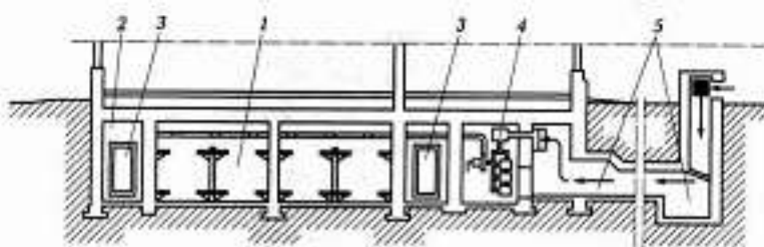
Рис. 1.2. Противорадиационное укрытие: 1 — отсеки для укрытых людей; 2 — тамбур; 3 — защитно-герметичные двери; 4 — фильтровентиляционная установка; 5 — аварийный выход, используемый для забора воздуха
