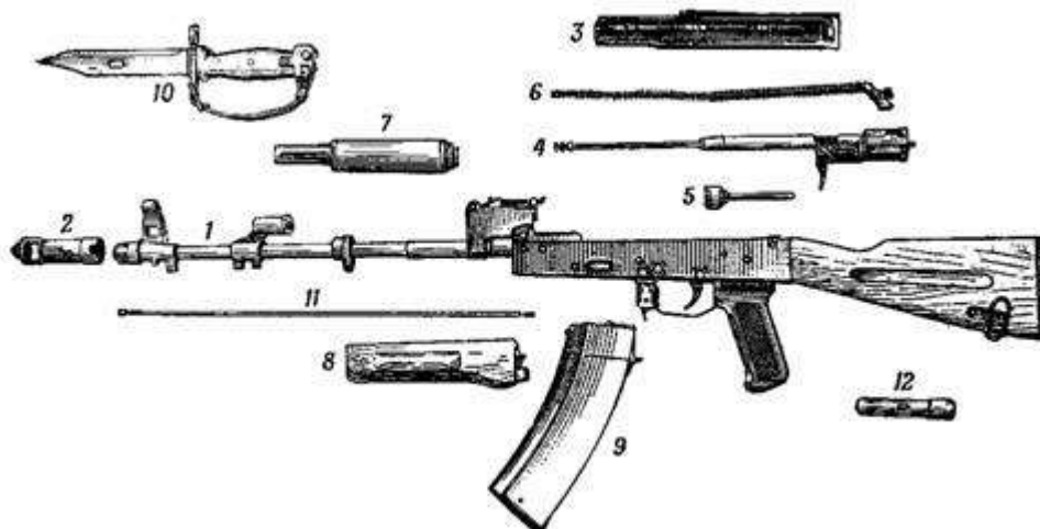
Общий вид 5,45-мм автоматы Калашникова
