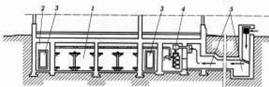
Рис. 1.2. Противорадиационное укрытие: 1 — отсеки для укрытия людей; 2 — тамбур; 3 — защитно-герметические двери; 4 — фильтровентиляционная установка; 5 — аварийный выход, используемый для забора воздуха
