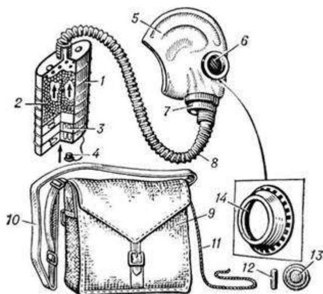
Рис. 2. Фильтрующий противогаз
