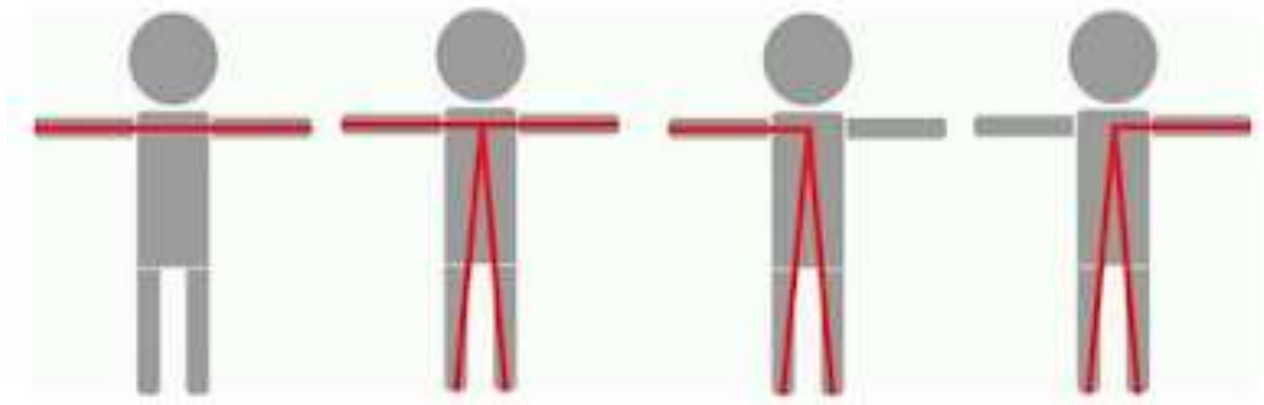
Рисунок 2. Наиболее опасные схемы прохождения электрического тока: рука-рука; руки-ноги; правая рука- левая и правая нога; левая рука и левая и правая нога
