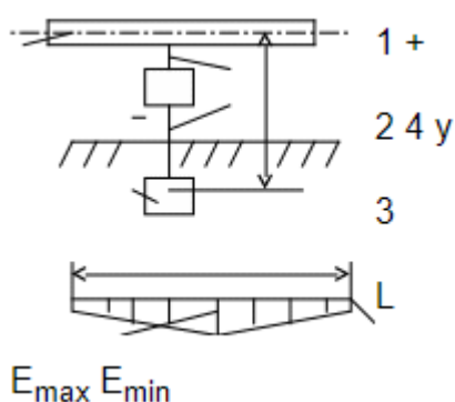
Рис. 2.1. Принципиальная схема катодной защиты
