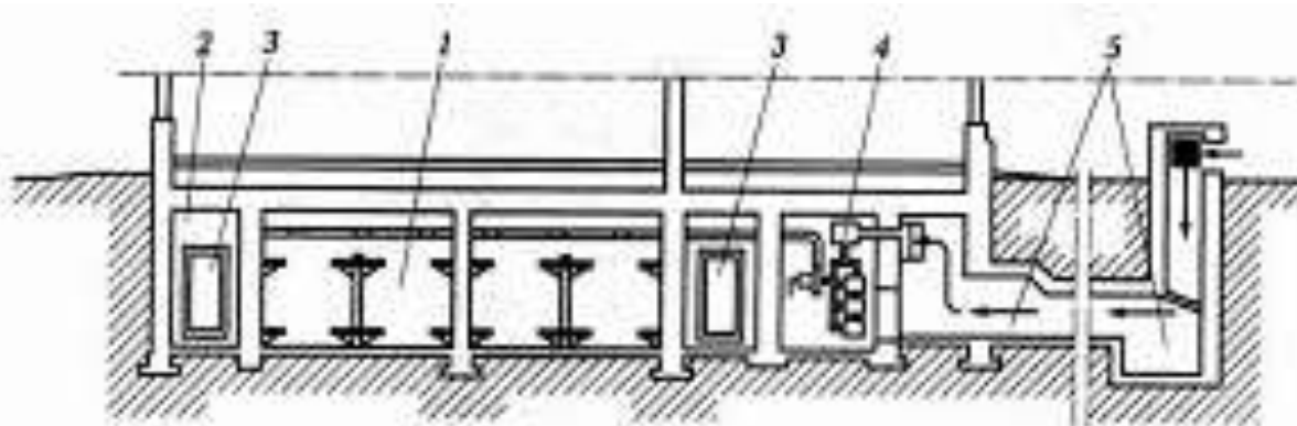
Рис. 1.2 Противорадиационное укрытие:
