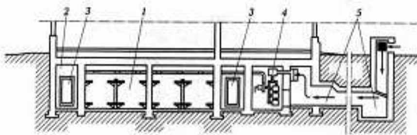
Рис. 1.2. Противорадиационное укрытие: 1 — отсеки для укрываемых людей; 2 — тамбур; 3 — защитно-герметические двери; 4 — фильтровентиляционная установка; 5 — аэриальный выход, используемый для забора воздуха
